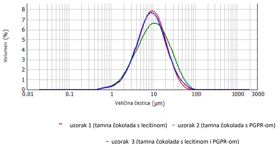
Slika 21 Prikaz veličine čestica tamnih čokolada s različitim emulgatorima
