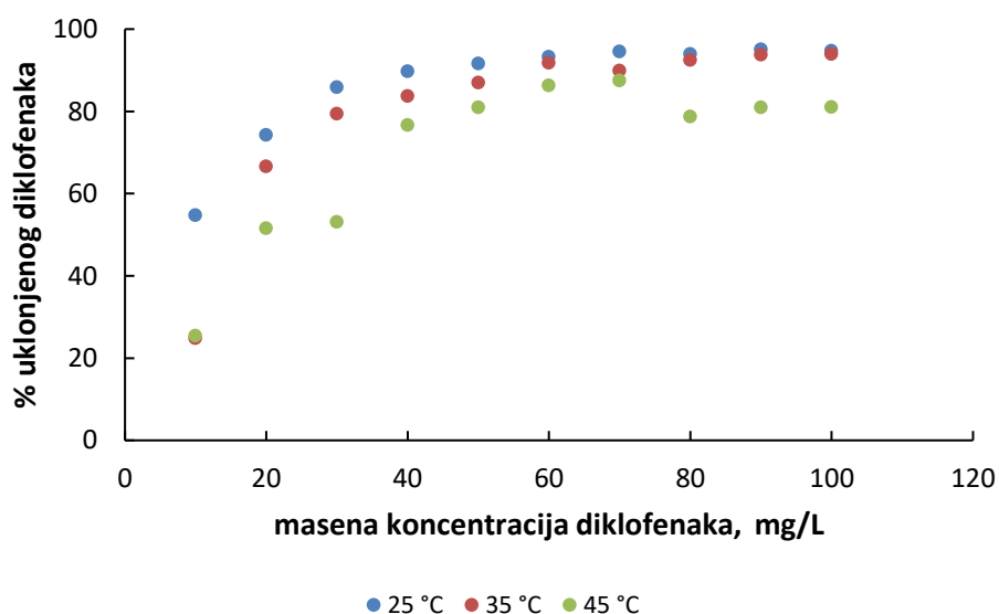
Slika 9 Utjecaj temperature na postotak uklanjanja diklofenaka iz modelnih otopina aktivnim ugljenom od ljuske oraha ( \gamma_{\text{diklofenak}} = 10, 20, 30, 40, 50, 60, 70, 80, 90 i 100 mg/l, V_{\text{otopine}} = 25 mL, m_{\text{adsorbensa}} = 0,1 g, rpm = 150/min, T=25, 35, 45 °C)
