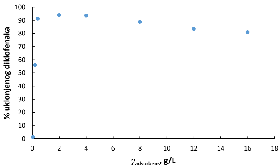
Slika 6 Uklanjanje diklofenaka iz vodenih otopina adsorpcijom na aktivni ugljen od ljuske oraha ( \gamma_{diklofenak} = 50 \text{ mg/L} , V_{otopine} = 50 \text{ mL} , \text{pH} = 5,5 , t = 360 \text{ min} , 150 \text{ rpm} , T = 25 \text{ °C} )
