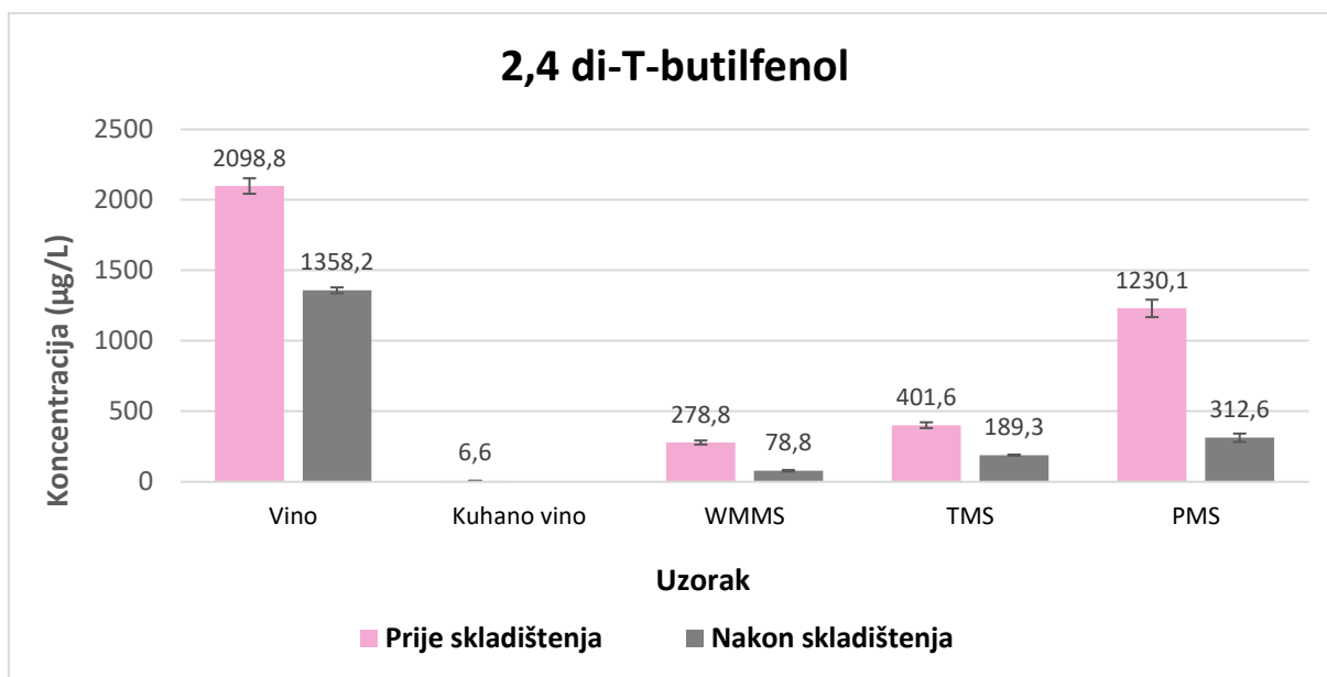
Slika 14 Sadržaj 2,4 di-T-butilfenola u početnom vinu, kuhanom vinu i kremama od vina s dodatkom modificiranih škrobova kukuruza (WMMS), tapioke (TMS) i krumpira (PMS) prije i nakon tromjesečnog skladištenja
