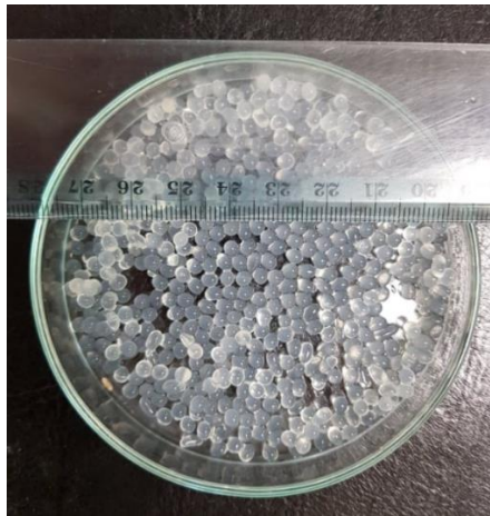
Slika 3.14. Kapsule alginata s imobiliziranim enzimom lakaza
