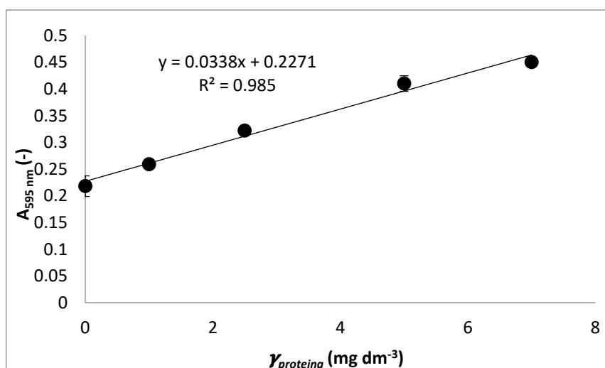
Slika 3.15. Kalibracijska krivulja za određivanje koncentracije proteina
