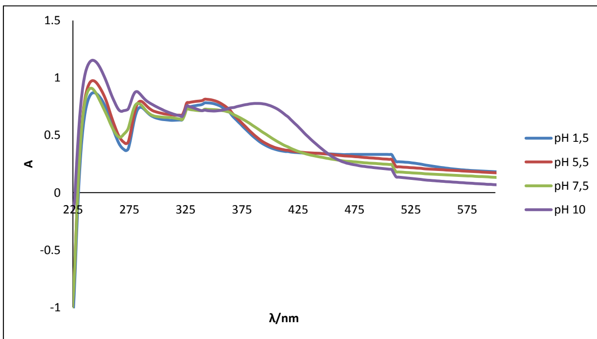
Slika 16 UV-Vis apsorpcijski spektar modela polifenola kore jabuke i β-glukana (5 mg L -1 ) u ovisnosti o različitoj pH vrijednosti pufera (5h)
