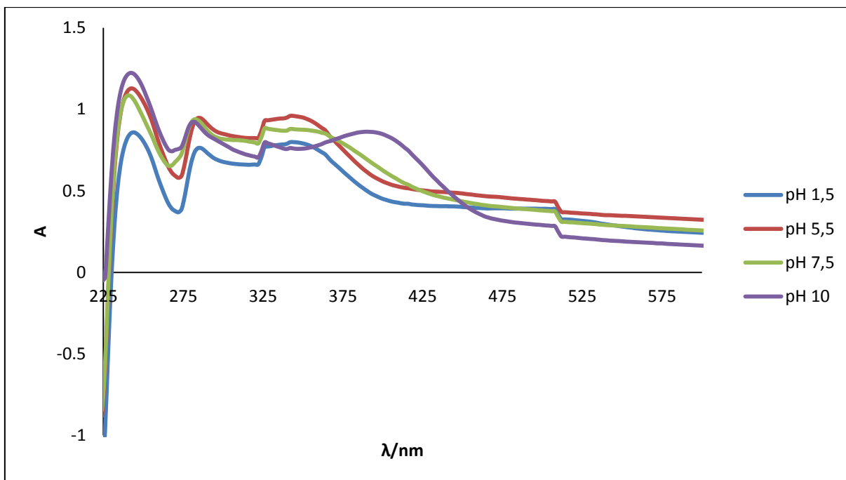
Slika 15 UV-Vis apsorpcijski spektar modela polifenola kore jabuke i β-glukana (5 mg L -1 ) u ovisnosti o različitoj pH vrijednosti pufera (2h)
