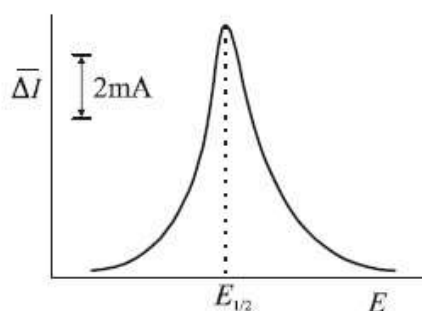
Slika 5 Izgled diferencijalnog pulsno voltamograma (Piljac, 2010)
