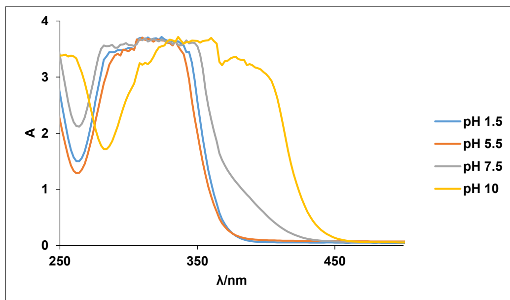
Slika 16 UV/Vis spektar otopine klorogenske kiseline (150 mg L -1 ) pri pH 1,5, 5,5, 7,5 i 10
