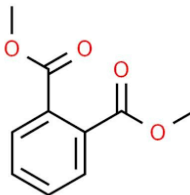
Slika 4. Kemijska struktura dimetil ftalata (Izvor: http://hr.alfachemar.com/organic-chemistry/dimethyl-phthalate-cas-no-131-11-3.html )
