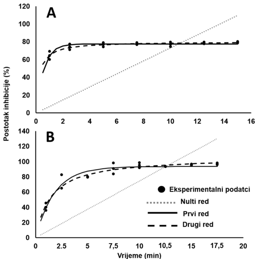
Slika 28 Nelinearna regresija eksperimentalnih podataka (% inhibicije enzima ukupnim polifenolima kožiće jabuke u ovisnosti o vremenu) jednadžbama nultog, prvog i drugog reda. A- \alpha -amilaza; B- \alpha -glukozidaza
