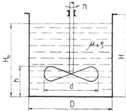
Slika 6. Karakteristične dimenzija miješala (Tomas i sur., 2013)
