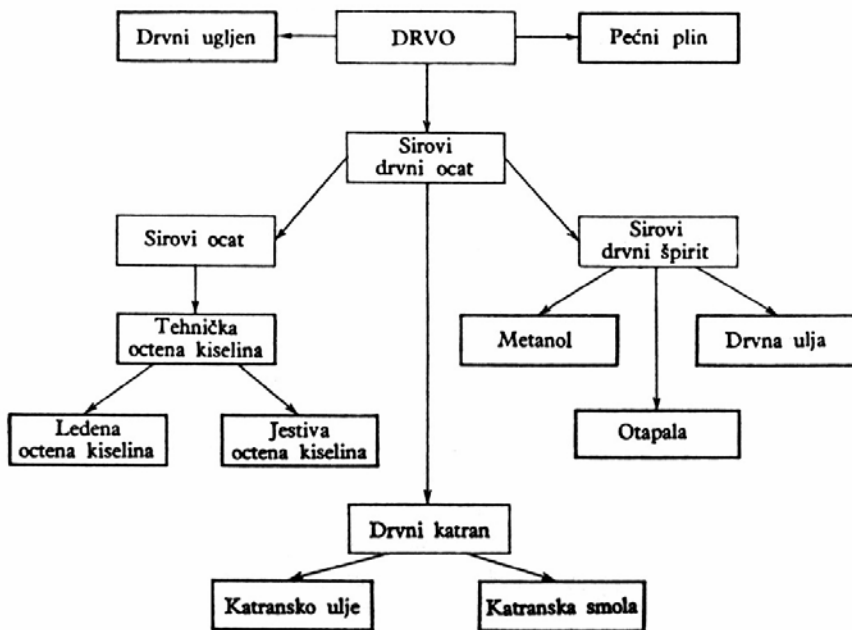
Slika 1. Osnovni proizvodi i poluproizvodi suhe destilacije drveta.
