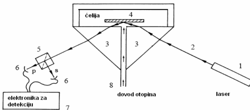
Slika 2. Shematski prikaz optičkog reflektometra: 1- He/Ne laser, 2- polarizirana zraka, 3- staklena prizma, 4- adsorbirajuća površina, Si/SiO 2 pločica, 5- razdjovnik zraka, 6- fotodioda, 7- računalo, 8- sustav za dovod otopina.
