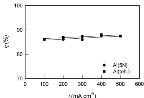
Slika 6. Ovisnost anodne djelotvornosti o primijenjenoj gustoći struje za čisti i tehnički Al u 2 \text{ mol dm}^{-3} NaCl otopini pri 25^\circ\text{C}
