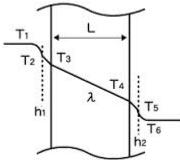
Slika 1 Prolaz topline s toplijeg na hladniji fluid kroz čvrstu stjenku (TLV, 2013)
