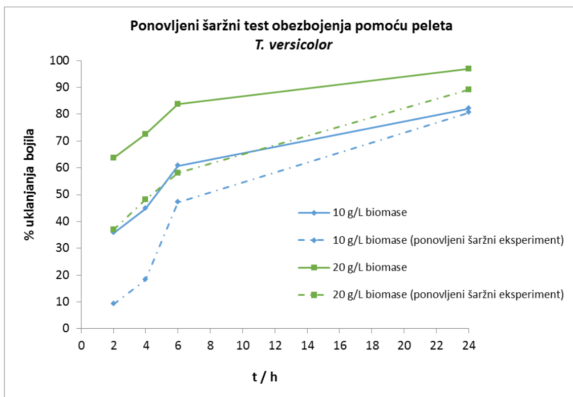
Slika 4.5. Ponovljivi šaržni test obezbojenja pomoću peleta T. versicolor ( T = 25^{\circ} \text{C} , n = 120 okr \text{min}^{-1} , \gamma_{\text{malahitno zelenilo}} = 5 \text{ mg L}^{-1} , \gamma_{\text{biomasa}} = 10 i 20 \text{ g L}^{-1} )
