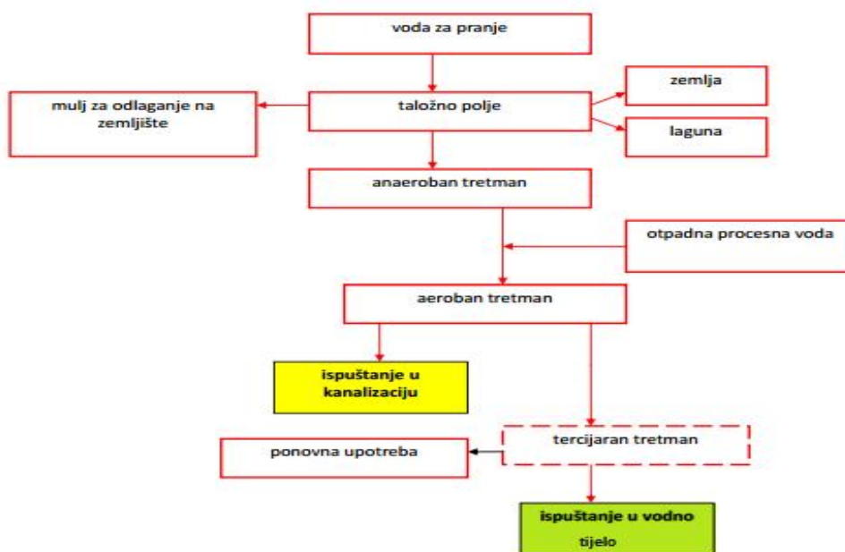
Slika 10 Procesni dijagram pročišćavanja otpadnih voda industrije šećera (Dalmacija, 2011)
