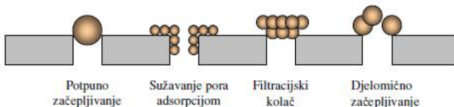
Slika 8 Mehanizam začepeljivanja (Mijatović i Matošić, 2008)
