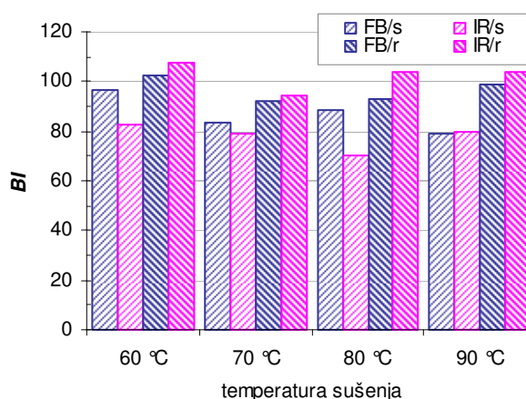
Slika 4.70 Vrijednosti indeksa posmeđivanja [ BI ] sušenih [s] i rehidratiranih [r] uzoraka mrkve (uzorak: M.III) u ovisnosti o temperaturi sušenja za dva različita načina sušenja (konvekcijsko u fluidiziranom sloju [FB], radijacijsko [IR])
