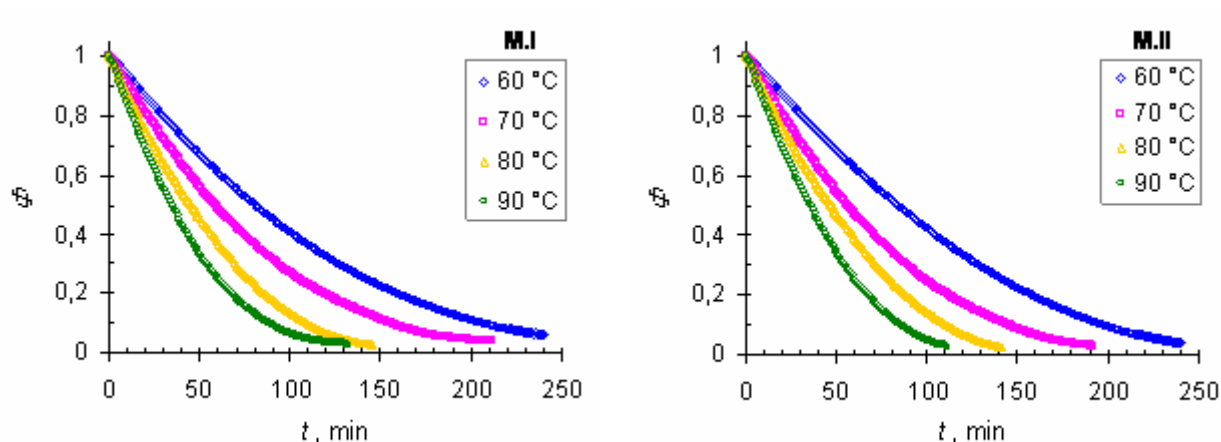
Slika 4.11 Eksperimentalni podaci infracrvenog sušenja mrkve (uzorci [M.I, M.II]) za različite temperature sušenja (ovisnost bezdimenzionalne vlažnosti [ \Phi ] o vremenu sušenja [ t ])
